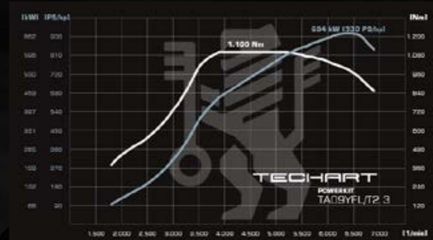
TECHART Power Kit TA 09YFL/T2.3 Cayenne Turbo GT E3.2 930 PS (684 kW), 1.100 Nm (+290 PS / 250 Nm) Nur für Rennsport / Export
