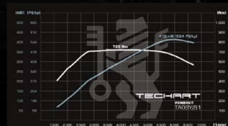
TECHART Power Kit TA 09YFL/S1 Cayenne S E3.2 564 PS (415 kW), 720Nm (+66 PS / 120 Nm) für Fahrzeuge mit/ohne OPF. Nur für Rennsport / Export
