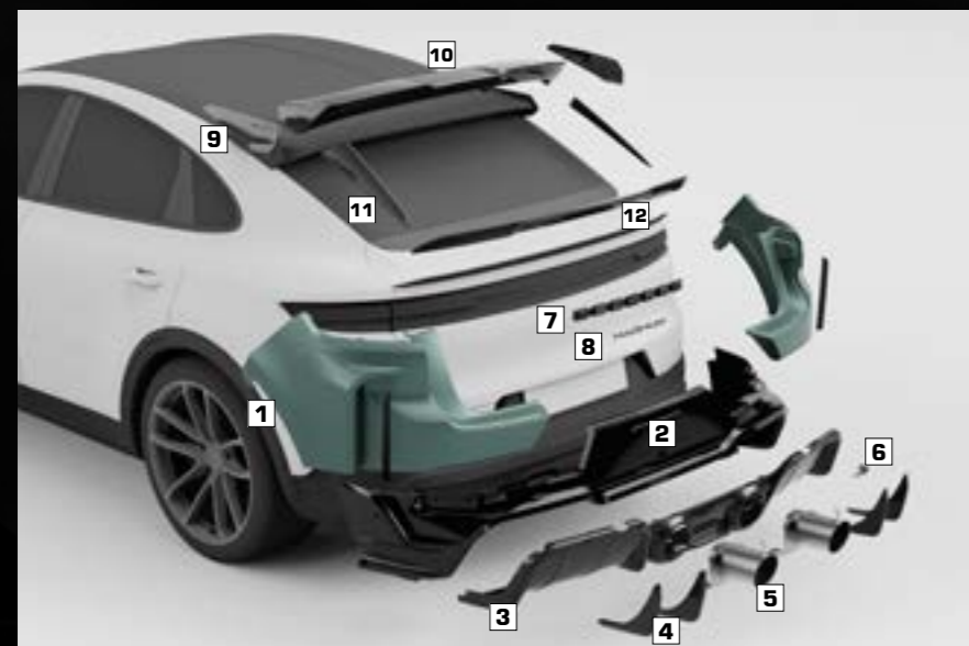
Aufbau MAGNUM Heckschürze zentrale Abgasanlage
