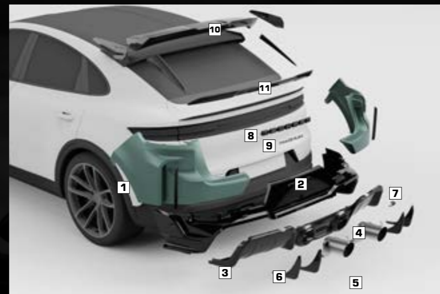
Aufbau MAGNUM Heckschürze seitliche Abgasanlage
