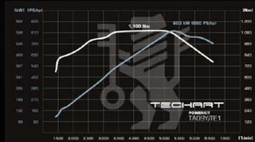
TECHART Power Kit TA 09YFL/TE1 Cayenne Turbo E-Hybrid E3.2 820 PS (603 kW), 1.100 Nm (+80 PS / 150 Nm) für Fahrzeuge mit OPF. Mit TÜV Gutachten
