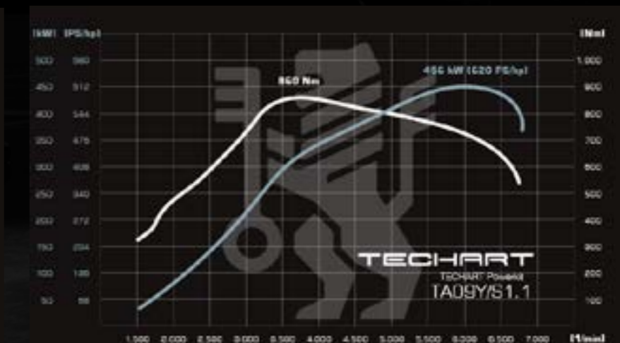
TECHART Power Kit TA 09YFL/S1.1 Cayenne GTS E3.2 620 PS (456 kW), 860 Nm (+120 PS / 200 Nm) für Fahrzeuge mit/ohne OPF. Nur für Rennsport / Export
