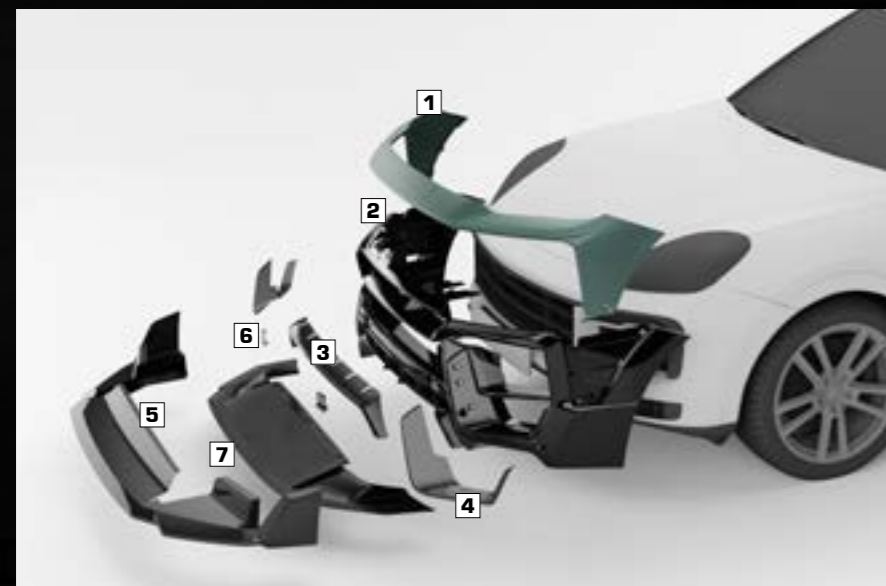
Aufbau MAGNUM Frontschürze
